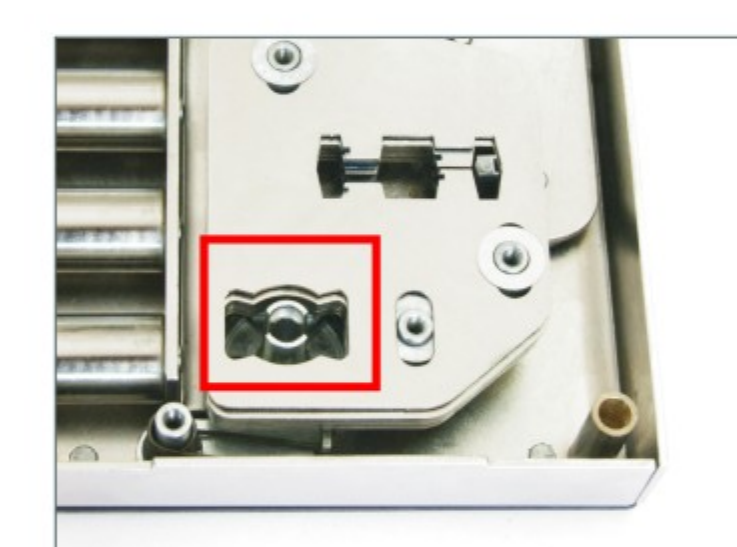
Сувальды оконного типа.
